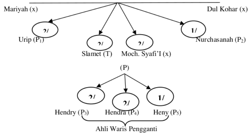
Gambar 1. Skema Pewarisan
